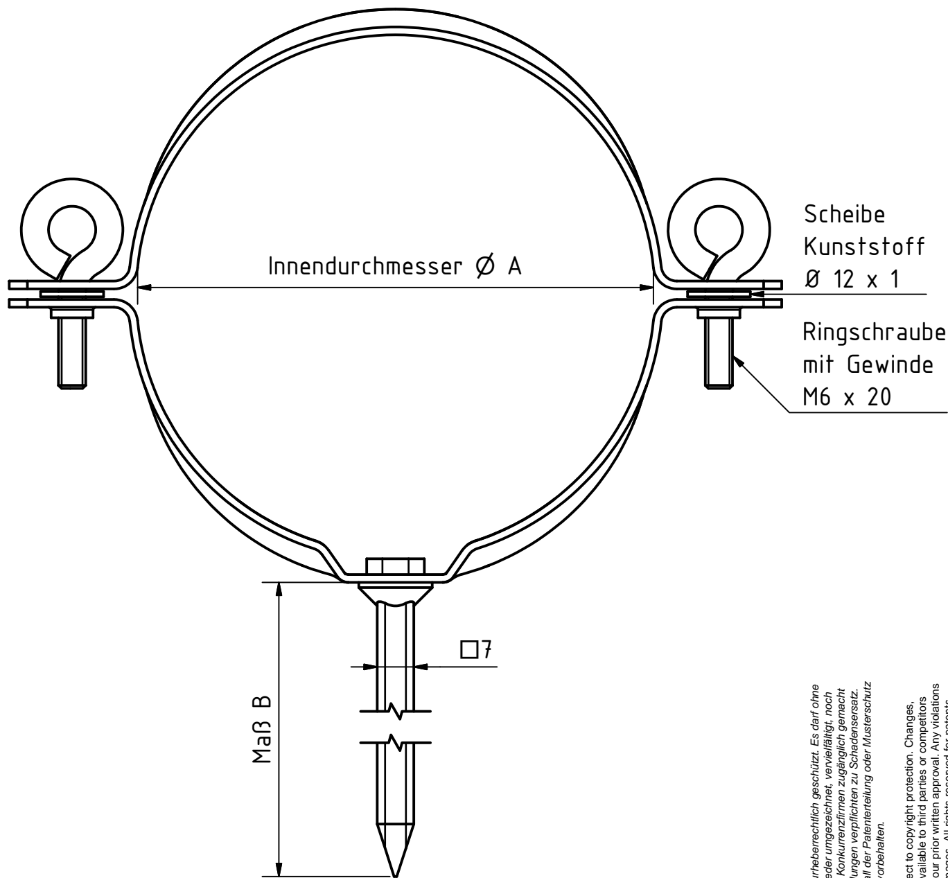
Draufsicht
